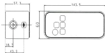
校正ユニット寸法図
