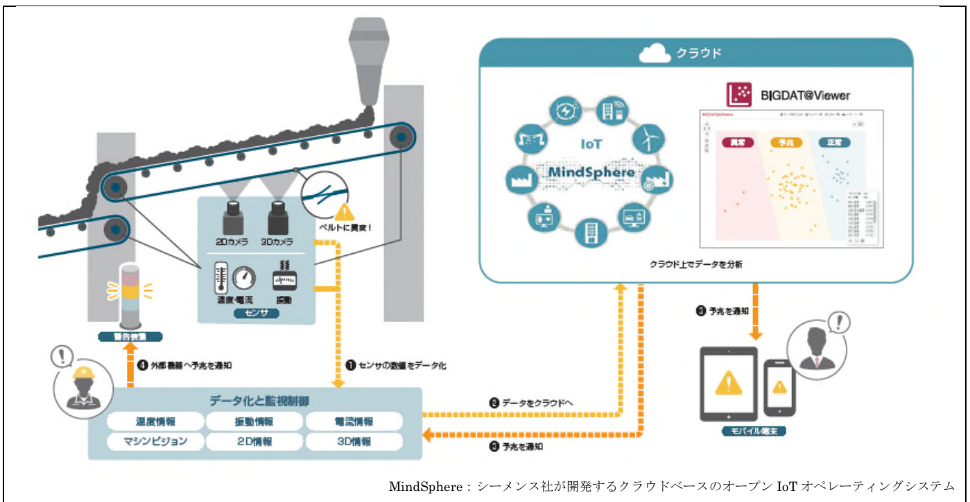
ベルトコンベア予知保全システムイメージ図
