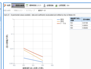
ひずみ寿命パラメータ (ε-N曲線)
