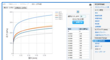
応力-ひずみ曲線データ
