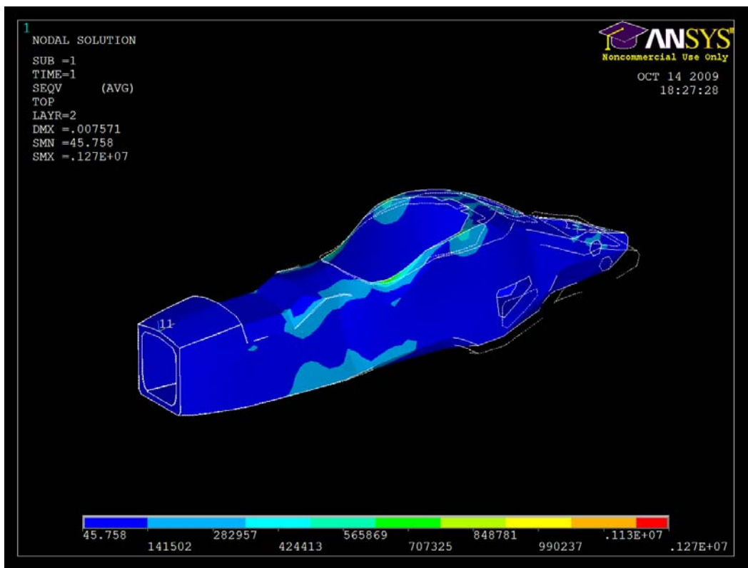
図5 . モノコックハニカム応力コンター ( Stress of Monocoque-honeycomb )
