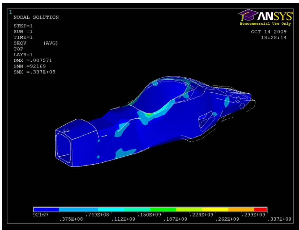
図6 . モノコックのインナー応力コンター ( Stress of inner-skin )
