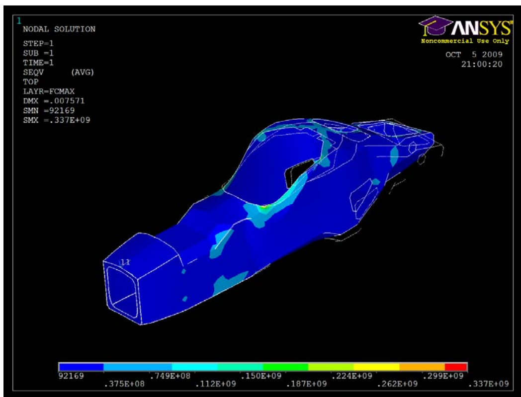
図4 . モノコックの OUTER 応力コンター ( Stress of outer-skin )
