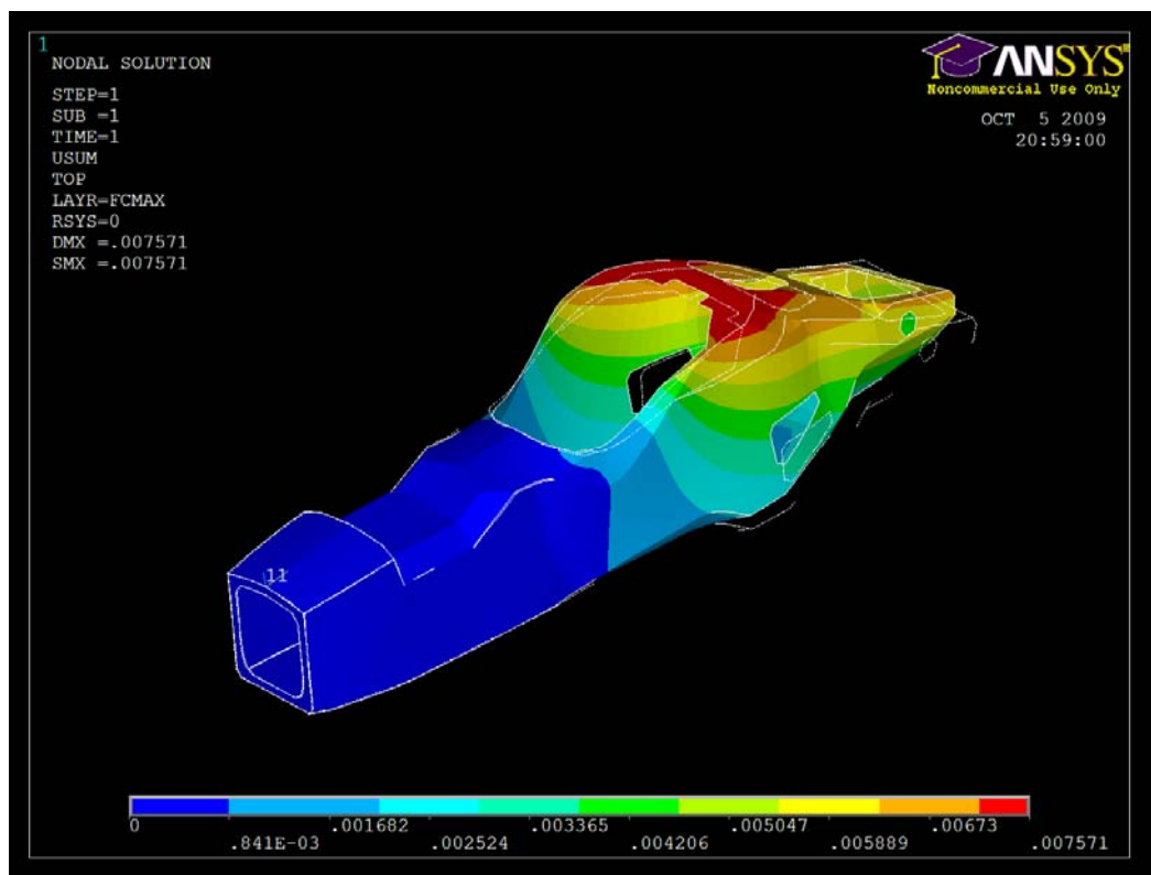
図3 . モノコックの変位コンター ( Deformation of Monocoque )
